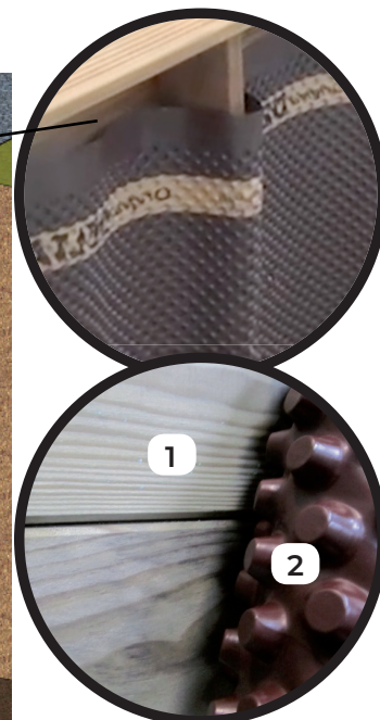
1- Armazón de composite 2- Rolo de protección y drenaje alveolar de PEHD
