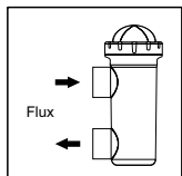
Le sens du fluide marqué sur la cellule doit être respecté. Le système de circulation doit garantir le débit minimal consigné dans le Tableau de Spécificités Techniques pour chaque modèle
