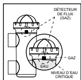
Le système détecteur de flux (détecteur de gaz) s'active en cas de non circulation de l'eau à travers la cellule ou bien si le flux est très faible. La non-évacuation du gaz d'électrolyse génère une poche qui isole électriquement l'électrode auxiliaire (détection électronique). Par conséquent, en introduisant les électrodes dans la cellule, la sonde de niveau (électrode auxiliaire) doit rester située dans la partie supérieure de celle-ci. La disposition la plus sûre est celle du diagramme d'installation recommandée.
