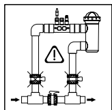
ATTENTION: le détecteur de flux ne fonctionnera pas correctement, ce qui produira un risque de rupture de la cellule, si les vannes d'entrée et de sortie de la canalisation où est installée la cellule d'électrolyse se ferment simultanément. Bien que cela reste une situation extrêmement inhabituelle, on peut l'éviter en bloquant, une fois l'équipement installé, la vanne de la sortie vers la piscine , de mode qu'elle ne puisse pas être manipulée accidentellement.
