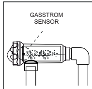
ALLOWABLE INSTALLATION ALLE MODELLE (Modelle 12/24/32 g/h mit Durchflusssensor)
