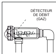
INSTALLATION AUTORISÉE TOUS LES MODÈLES (Modèles 12/24/32 gh avec capteur de débit)
