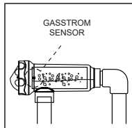
ZULÄSSIGE INSTALLATION ALLE MODELLE (Modelle 12/24/32 LS g/h mit Durchflusssensor)
