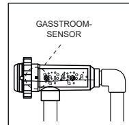
INSTALLATIE TOEGESTAAN ALLE MODELLEN (Model 12/24/32 LS g/u met flowsensor)
