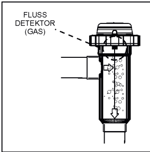
Abb. 5 EMPFOHLENE Installation
