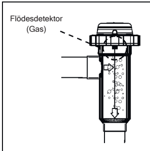
Fig. 5 REKOMMENDERAD installation
