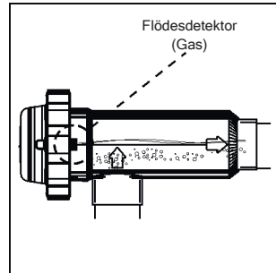
Fig. 6 GODTAGBAR installation
