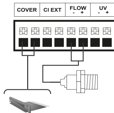
③ Induktiver Durchflussmesser
