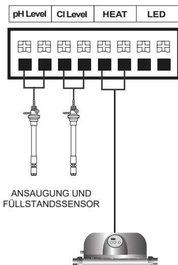
④ Füllstandssensor
