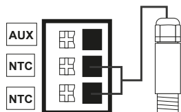
① Temperatursensor
