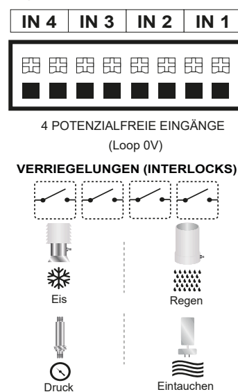
⑦ Verriegelungen (Interlocks)
