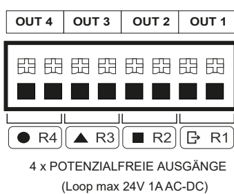
⑤ Ausgänge R1-R4
