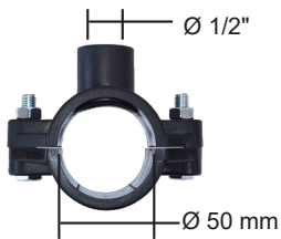
Manschette
