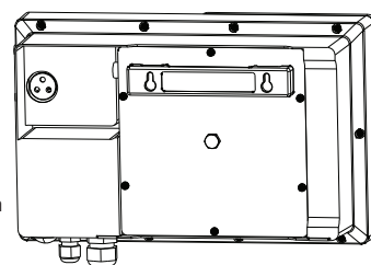
Instalace zařízení na stěnu
