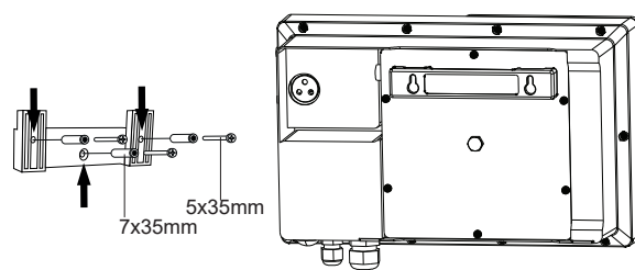
A berendezés falra szerelése
