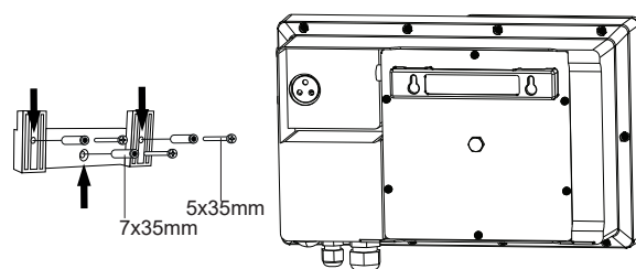
Montaż natynkowy urządzenia
