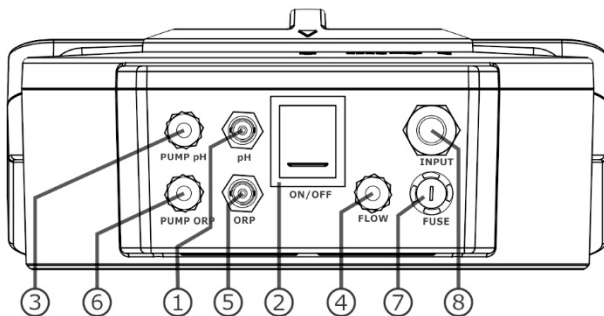
Abb. 4. Bedienfeld des UV LP/LP+ Systems Rückansicht
