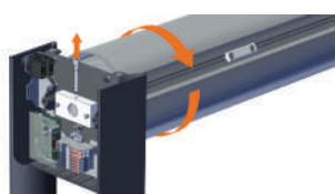
Moteur débrayable
