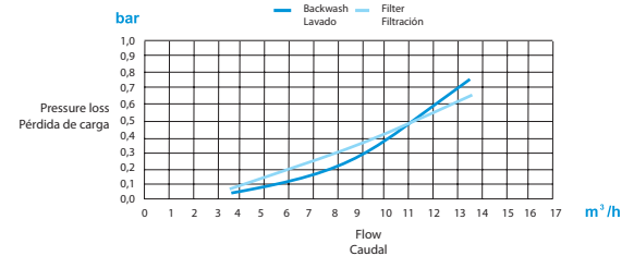
Valve 1 1/2" Válvula 1 1/2"
