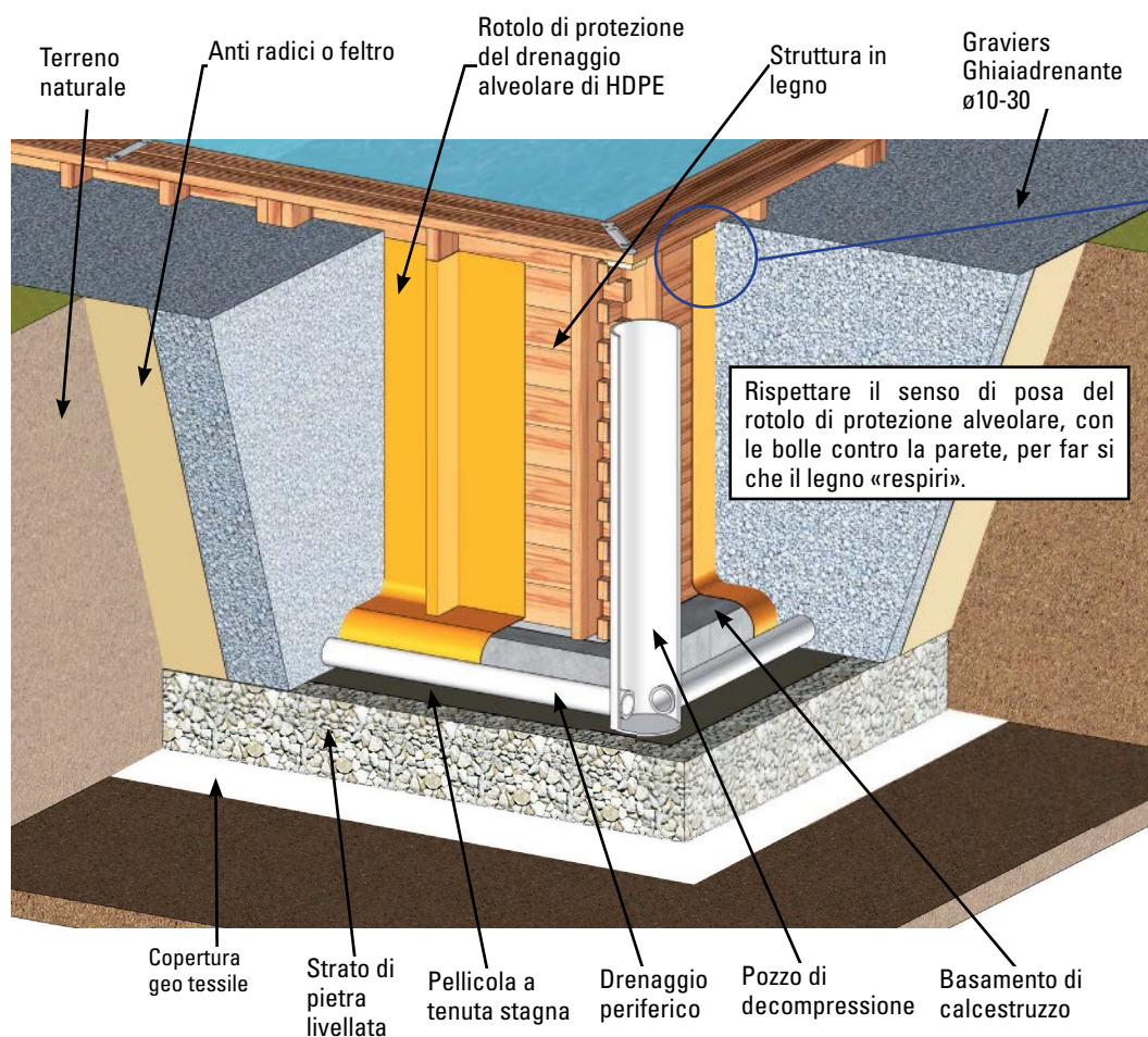
1- Struttura in legno 2- Rotolo di protezione del drenaggio alveolare di HDPE
