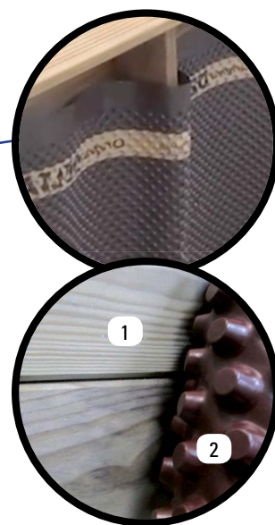
1- Struttura in legno 2- Rotolo di protezione del drenaggio alveolare di HDPE
