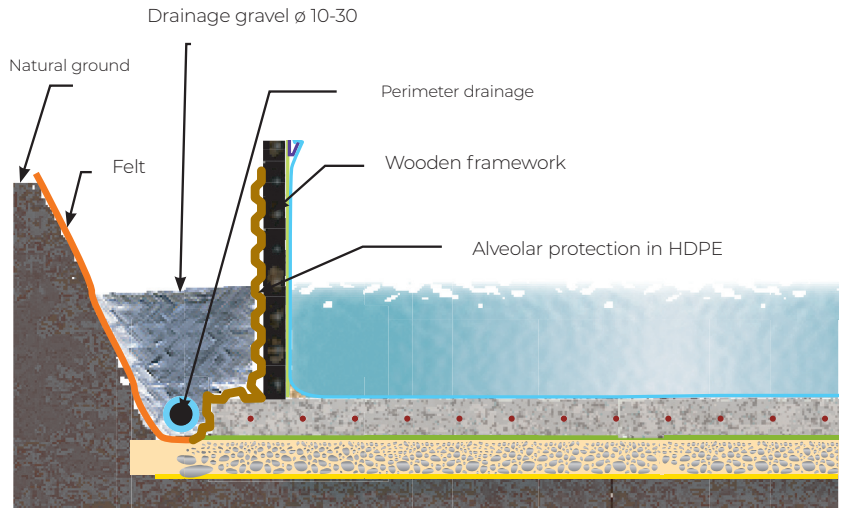
Alveolar protection layer HDPE
