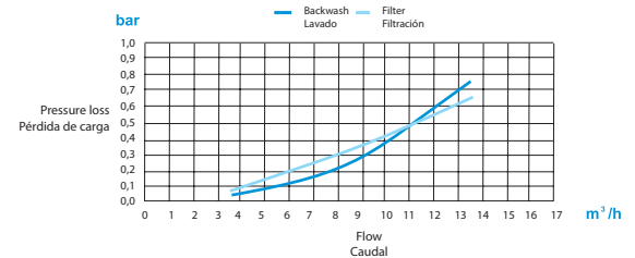
Valve 1½" Válvula 1½"
