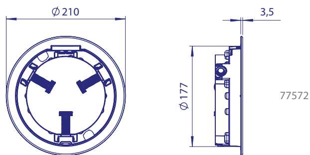
Flexi siering voor betonnen zwembaden
