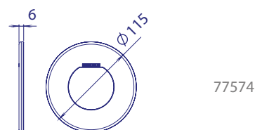
FlexiMini afwerkingsring voor beton of polyester zwembaden
