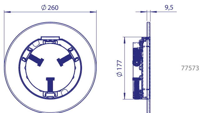
Flexi afwerkingsring voor liner zwembaden of bestaande betonnen zwembaden
