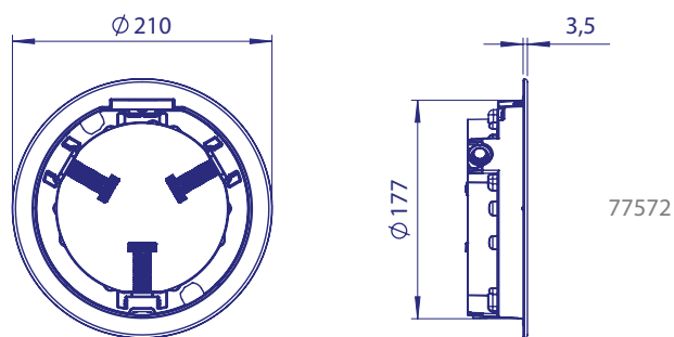
Embelledor Flexi para piscinas de hormigón
