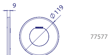
Embelledor FlexiMini para piscinas de liner
