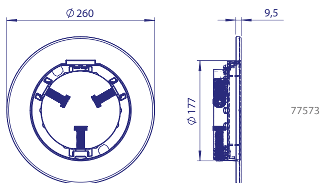
Embelledor Flexi para piscinas de liner o existentes de hormigón
