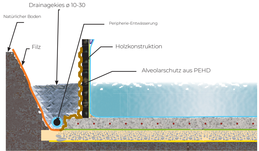
Alveolarschutz aus PEHD
