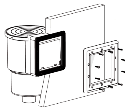
Montage der ersten Skimmerdichtung
