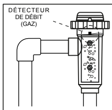
Installation RECOMMANDÉE
