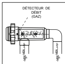
Installation ADMISE (Avec installation du flussostat)
