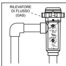
Installazione CONSIGLIATA
