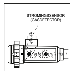
NIET-AANVAARDBARE installatie
