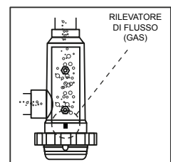
Installazione NON AMMESSA
