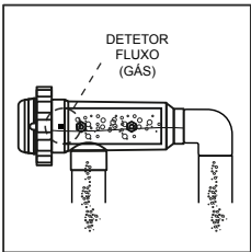
Instalação PERMITIDA (Junto à instalação do fluxostato)
