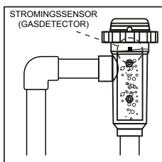
AANBEVOLEN installatie
