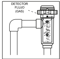
Instalación RECOMENDADA
