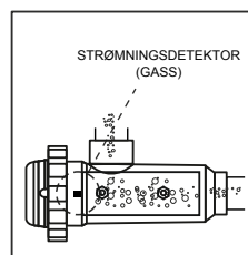
UAKSEPTABEL installasjon
