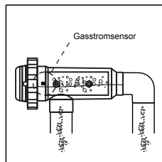
ZULÄSSIGE Installation (Neben der Installation des Durchflussschalters)
