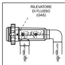
INSTALLAZIONE CONSENTITA (Accanto all'installazione del flussostato)
