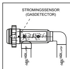
TOEGESTANE installatie (Naast installatie van de flowschakelaar)
