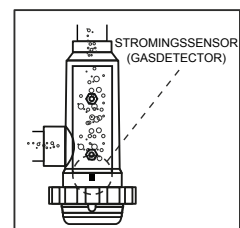
NIET-AANVAARDBARE installatie
