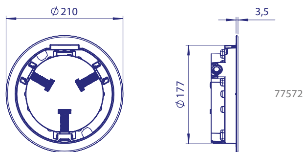
Embelezador FlexiPure para piscinas de betão
