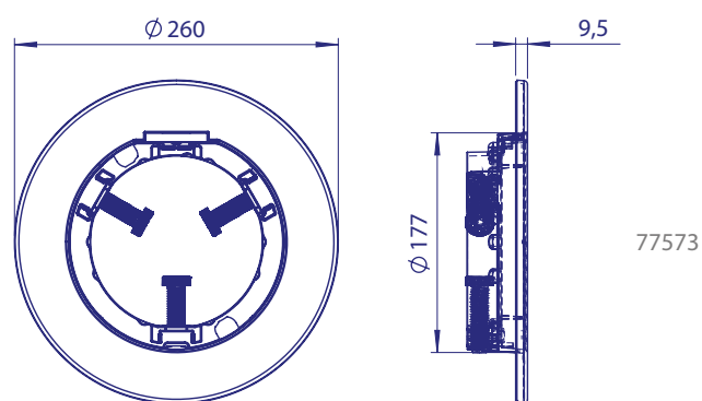
Embelezador FlexiPure para piscinas de liner ou de betão já existentes
