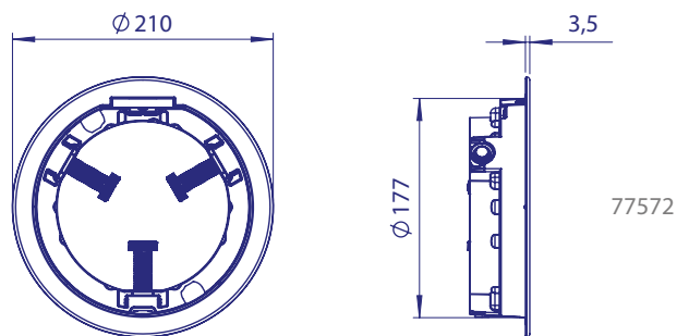
Cache FlexiPure pour piscines en béton
