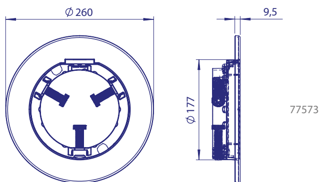
Cache FlexiPure pour piscines en liner ou en béton existantes
